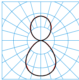
Lunexo H1 CDP-I 6500 840 +LLWM 01 TX050910
