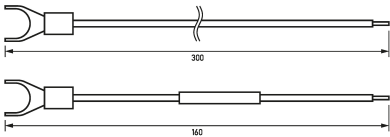
Maßzeichnung Gruppenansicht
