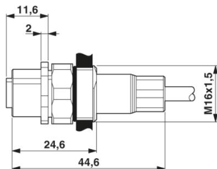
M12-Einbausteckverbinder
