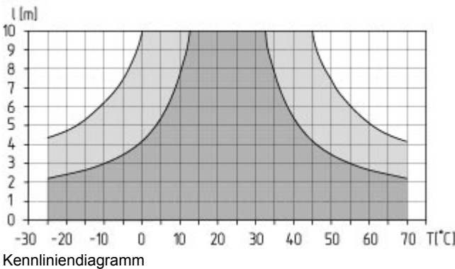
Kennliniendiagramm
