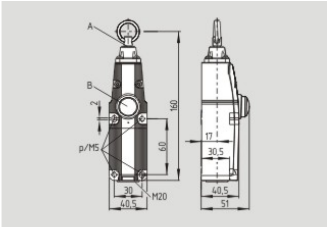
Maßzeichnung (Grundgerät)
