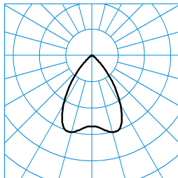
InperiaL G2 C07 BR19 1000-840 01 + RD-PC ■ C0 - C180 TX37381
