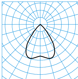
InperiaL G2 C07 BR19 1000-840 01 ■ C0 - C180 TX372371
