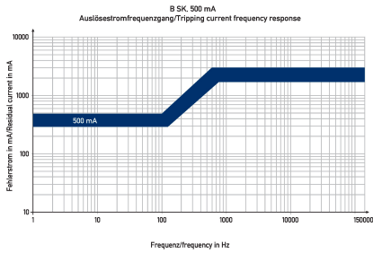
Kennlinie B SK 500 mA
