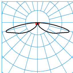
LTX LT-SB3L-LRA/1500-740 2G1 TX084136
