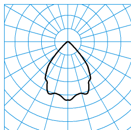
InperiaLP C05 HR22 1800-940 01 + ZN-PC ■ C0 - C180 TX373663
