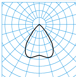
InperiaL G2 C07 BR19 2700-830 01 ■ C0 - C180 TX373223
