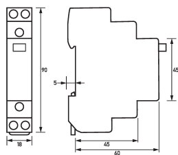
Maßzeichnung Gruppenansicht
