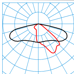
Cuvia 40-AB2L-LRA/3200-740 4G1S TX046958
