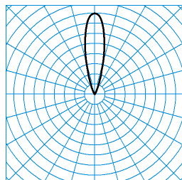
Altigo G2 60 RM3L/2000-830 1G1P + G2 VE IP66 24V DC 30W ■ C0 - C180 TX113950 DIN 5040: E04 UTE: 0,00 J + 1,00 T CEN Flux Code: 0 0 0 0 100 97 99 100 100
