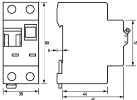
Maßzeichnung Gruppenansicht
