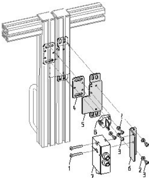
Produktgrafik (Explosionszeichnung)
