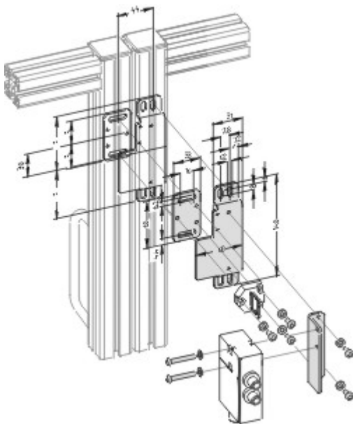
Maßzeichnung (Sonstige)
