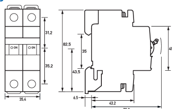
Maßzeichnung Gruppenansicht
