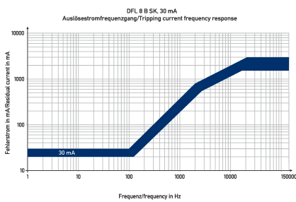
Kennlinie B SK 30 mA
