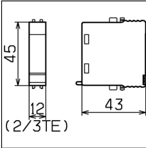
Maßbild BCT MLC BE
